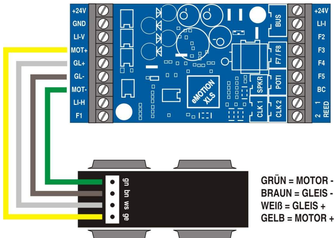
Abbildung 4: Anschluss an LGB® Getriebe
