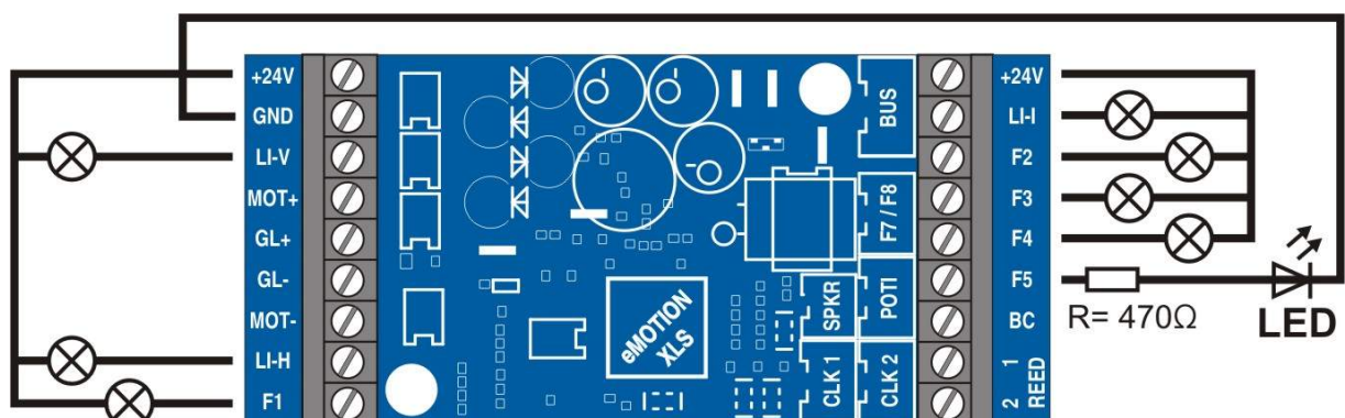
Abbildung 9: Licht und Funktionsausgänge und deren Verschaltung
