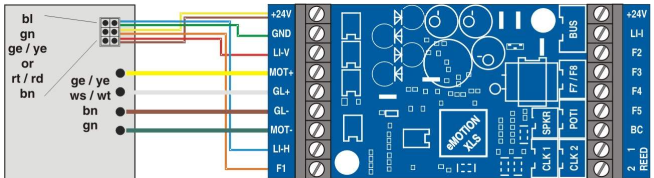
Abbildung 6: Einbau in Lok mit LGB® Dekoder-Schnittstelle
