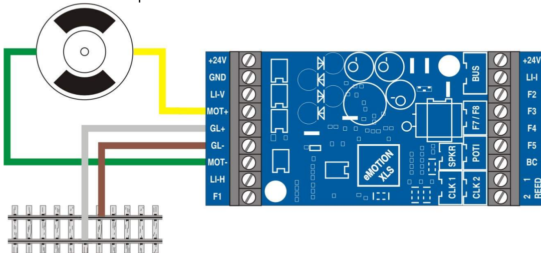
Abbildung 3: Einbau des eMOTION XLS
