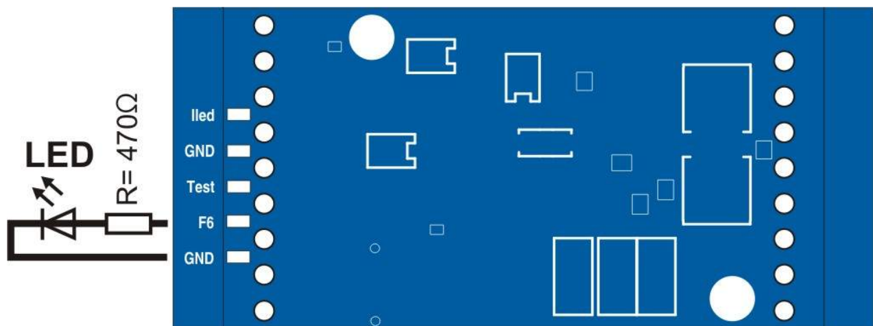
Abbildung 10: Licht und Funktionsausgang Unterseite und dessen Verschaltung
