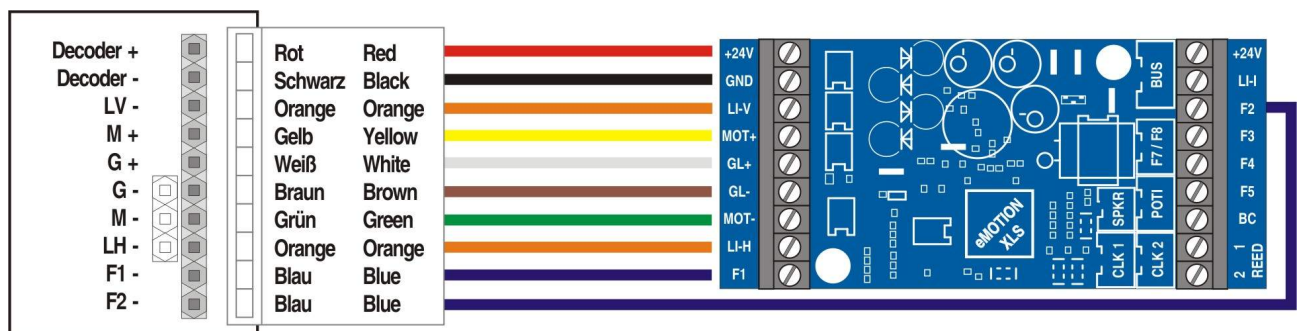
Abbildung 7: Verwendung des Schnittstellenkabels an LGB® DCC Schnittstelle
