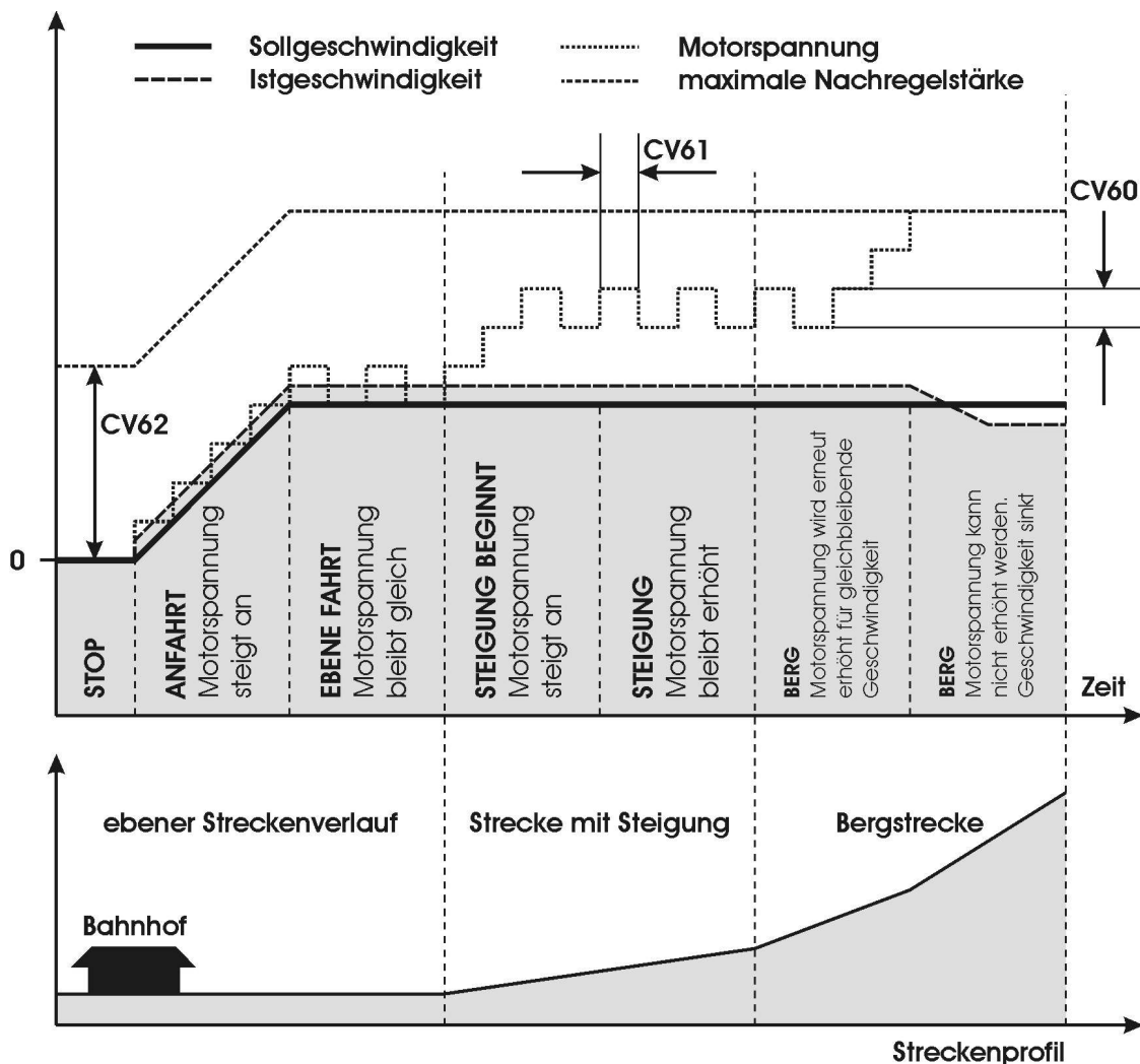
Abbildung 13: Funktionsweise der Lastregelung
