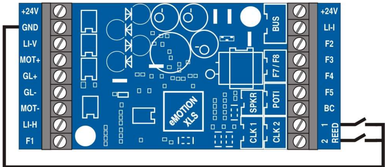
Abbildung 11: Anschluss der Reedkontakte
