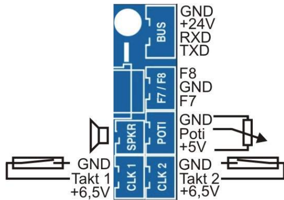
Abbildung 2: Belegung der Anschlussbuchsen
