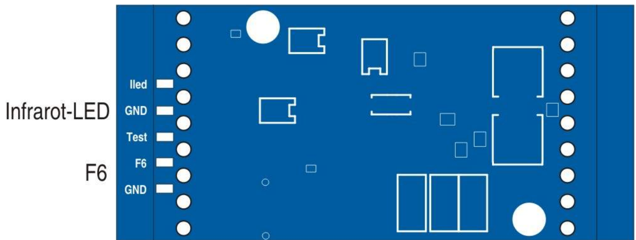
Abbildung 5: Belegung der Anschlusslötkontakte (Unterseite)
